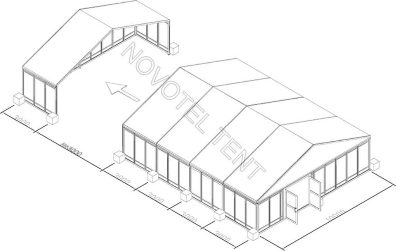
诺沃特篷房NST系列10米跨度篷房效果示意图
