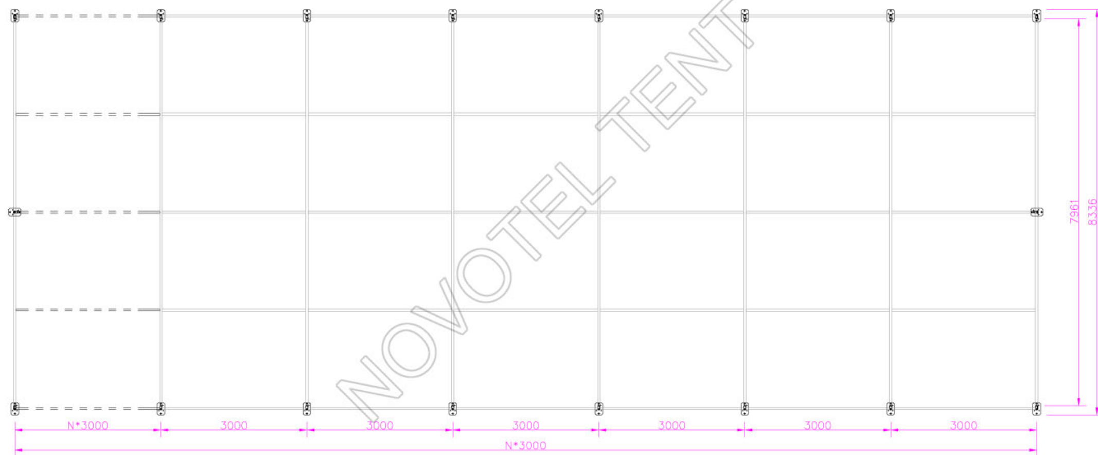
跨度8m*长度【N*3m】平面布局
