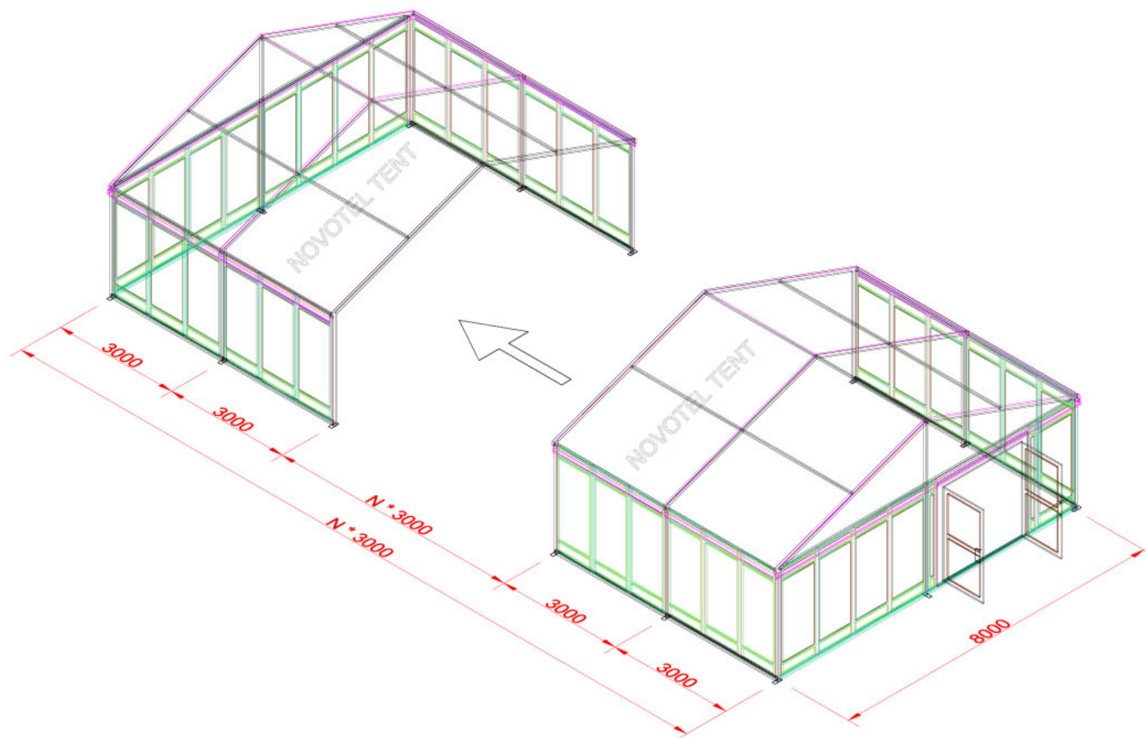
诺沃特篷房NST系列8米跨度3D结构示意图标注
